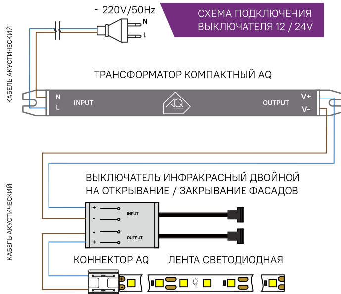
СХЕМА ПОДКЛЮЧЕНИЯ ВЫКЛЮЧАТЕЛЯ 12 / 24V
