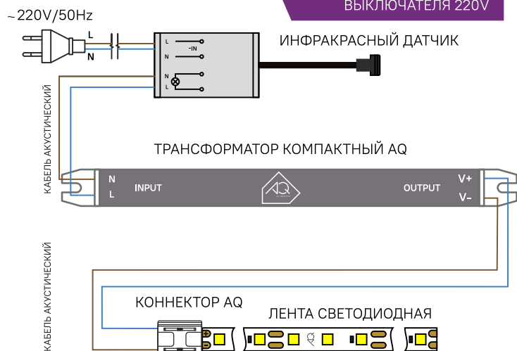
СХЕМА ПОДКЛЮЧЕНИЯ ВЫКЛЮЧАТЕЛЯ 220V
