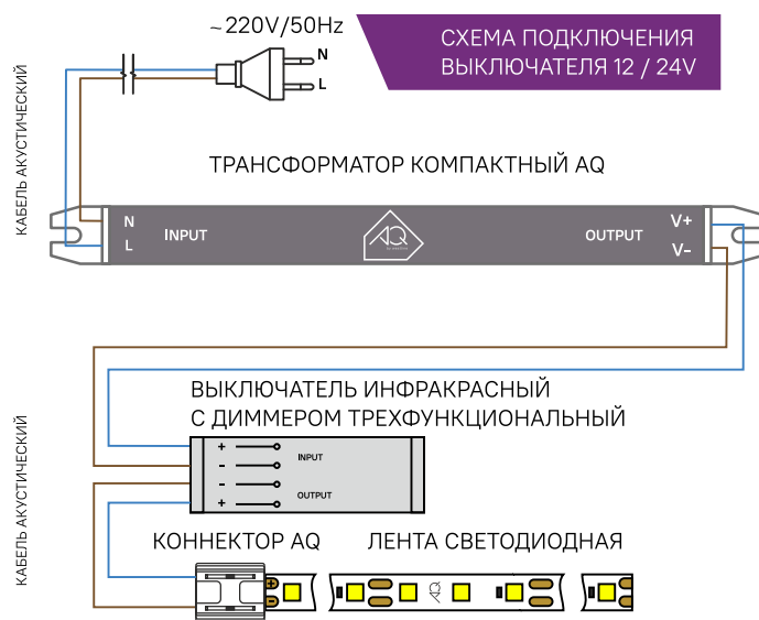
СХЕМА ПОДКЛЮЧЕНИЯ ВЫКЛЮЧАТЕЛЯ 12 / 24V
